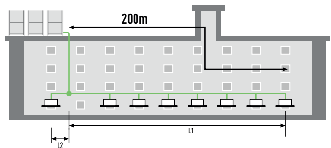
L1 = Längster Rohrleitungsstrang, L2 = Kürzester Rohrleitungsstrang, L1 - L2 = max. 50 m
